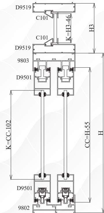
MẶT CẮT 1:1
