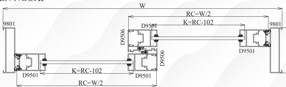
MẶT CẮT 2:2
